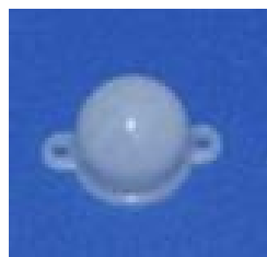
型号: 2136-1 尺寸: 23.8 \times 16.3 \times 13.1 焦距: 7.5mm 感应角度: 120^\circ 感应距离: 5m
