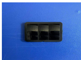
型号:YY-DL30 尺寸: 30.4*20.4 焦距: 35mm 感应角度: 30° 感应距离: 35-40m
