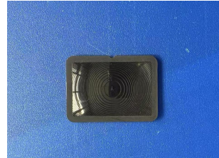
型号:YY-DL-50M 尺寸: 35*25 焦距: 50mm 感应角度: 3.5° 感应距离: 50m
