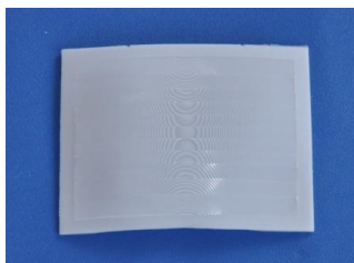
型号: 7809-2 尺寸: 56.3*43.7 焦距: 25mm 感应角度: 100° 感应距离: 12m
