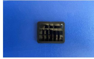
型号:YY-DL60 尺寸: 37.4*20.4 焦距: 25mm 感应角度: 60° 感应距离: 25-30m
