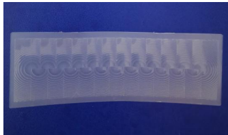
型号: YY-7526-25 尺寸: 74.82*25.7 焦距: 25mm 感应角度: 180° 感应距离: 18m
