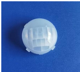
型号:YY-2311 尺寸: Ø23.22*12 焦距: 11mm 感应角度: 120° 感应距离: 10m 无纹区朝下, 放置 1.2m, 可防宠
