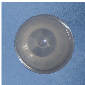
型号: 7709-4 尺寸: \phi 23.7*12.9 焦距: 11mm 感应角度: 120° 感应距离: 10m
