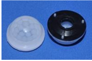
型号: 023115 尺寸: \varnothing 26 \times 17.3 焦距: 11.5mm 感应角度: 120^\circ 感应距离: 10m
