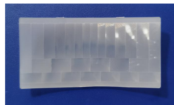
型号: YY-3468 尺寸: 34*68 焦距: 25mm 感应角度: 150° 感应距离: 15m
