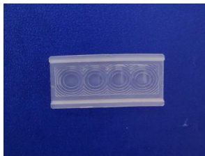
型号: YY-2312 尺寸: 12*23.5 焦距: 10mm 感应角度: 80^\circ 感应距离: 10m
