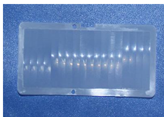
型号: 7707-B 尺寸: 39.5*85.3 焦距: 25mm 感应角度: 180° 感应距离: 16m
