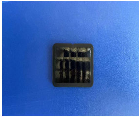
型号:YY-DL45 尺寸: 30.4*20.4 焦距: 25mm 感应角度: 45° 感应距离: 25-30m
