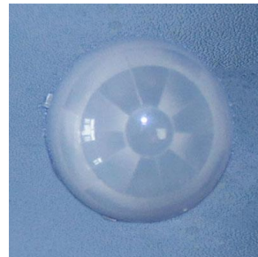
型号:PN-08-4G 尺寸: 15.21*14.95*5.48 焦距: 4mm 感应角度: 90° 感应距离: 3m
