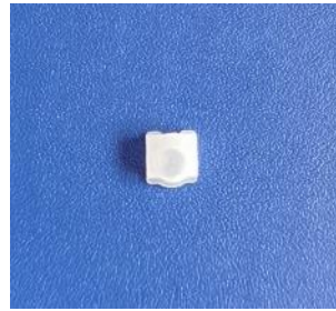
型号:XH-01 尺寸: 5.56*2.5 焦距: 2mm 感应角度: 90° 感应距离: 2m
