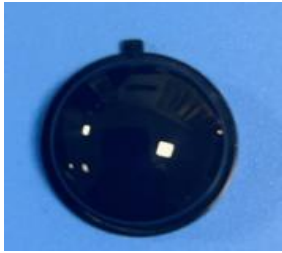
型号: 13120F-4 尺寸: \Phi 14.2 焦距: 6mm 感应角度: 120^\circ 感应距离: 6m
