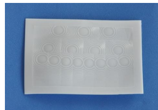
型号: 7703-1 尺寸: 61*42.7 焦距: 30.5mm 感应角度: 83° 感应距离: 15m
