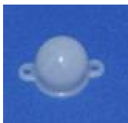
型号: 2136-1 尺寸: 23.8*16.3*13.1 焦距: 7.5mm 感应角度: 120 ° 感应距离: 6m
