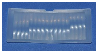
型号: 7707-1A 尺寸: 91.3*39.5 焦距: 25mm 感应角度: 180° 感应距离: 16m
