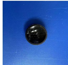
型号:YY-3012 尺寸: \varnothing 33.4 焦距: 12mm 感应角度: 120^\circ 感应距离: 12m
