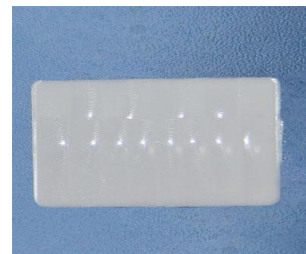
型号: 8202-1 尺寸: 38.2*21.5 焦距: 16mm 感应角度: 120° 感应距离: 12m
