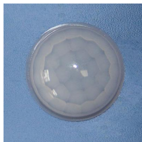
型号: 8003-2F-X 尺寸: 25.5*12.3 焦距: 10.5mm 感应角度: 120° 感应距离: 10m
