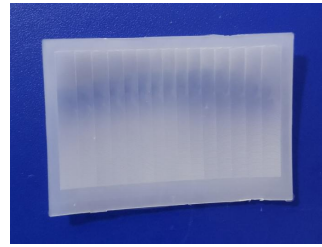
型号: YY-AA-12-V1 尺寸: 42.6*61 焦距: 30.5mm 感应角度: 100° 感应距离: 12m
