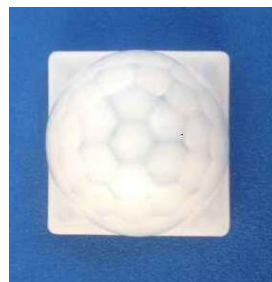
型号: 024120 去腿 尺寸: 23.57*23.5*17.2 焦距: 12mm 感应角度: 120° 感应距离: 12m
