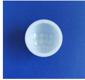
型号:YY-023115-15 尺寸: \Phi 26 焦距: 11.5mm 感应角度: 120^\circ 感应距离: 半径 10m
