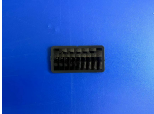
型号:YY-DL90 尺寸: 45.4*20.4 焦距: 25mm 感应角度: 90° 感应距离: 25-30m
