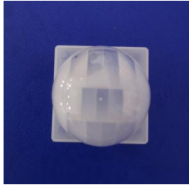
型号: YY-1003-45 尺寸: 24*24 焦距: 12mm 感应角度: 120^\circ 感应距离: 10m
