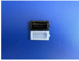
型号: YY-3015-8 尺寸: 30*15.7*0.8 焦距: 8mm 感应角度: 110° 感应距离: 8-10m
